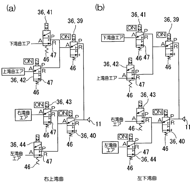
電磁弁を6コ用いた4方向の回路図 右上・左下の2方向の動き(右下・左上も同様)
